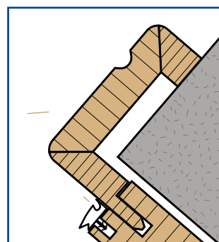
NORMZARGE MIT PROFILIERUNG
