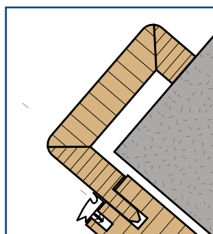
NORMZARGE MIT RUNDKANTE
